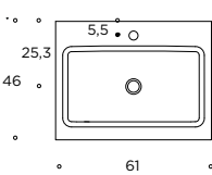
THIN 71 Art. A147 - P. 390 Lavabo consolle H 1,2 cm (con foro troppo pieno) Console washbasin H 1,2 (with overflow) Lavabo consolle H 1,2 (avec trop-plein)
