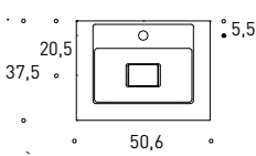
PAROS 71 Art. A887 - P. 386 Lavabo consolle H 1,5 cm (senza foro troppo pieno) Console washbasin H 1,5 (without overflow) Lavabo consolle H 1,5 (sans trop-plein)
