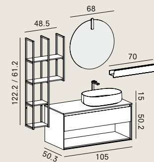
Face 01 L 105.6 cm × P 50.5 cm p — 02 PE1 pet bianco (L 205 cm con sporgenza mensola e pensili)
