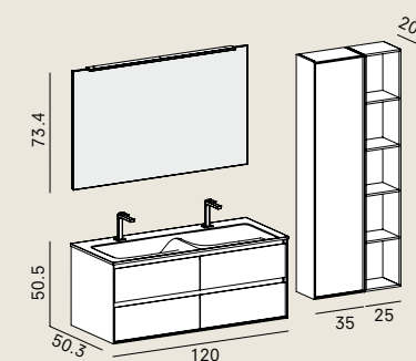
Face 05 L 121 × P 50.8 cm p — 28 PE3 pet fango
