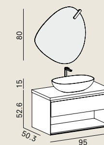
Face 06 L 95.2 × P 51 cm p — 36 PE3 pet fango
