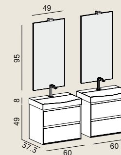
Face 02 L 61 × P 38/43 cm p — 10 PE2 pet visone
